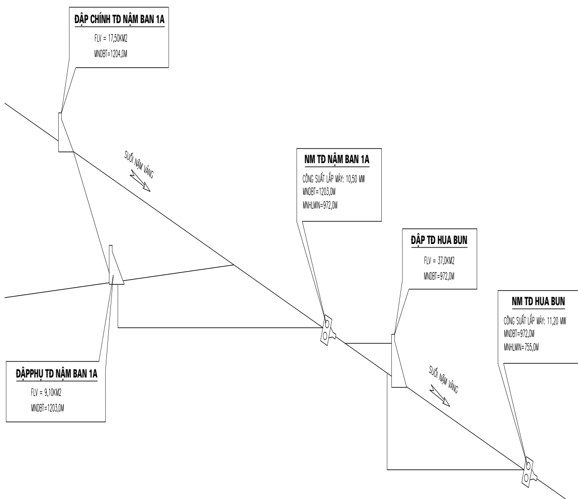
Hình 0. 1. Mối liên hệ quy hoạch thủy điện trên suối Nậm Vắng
