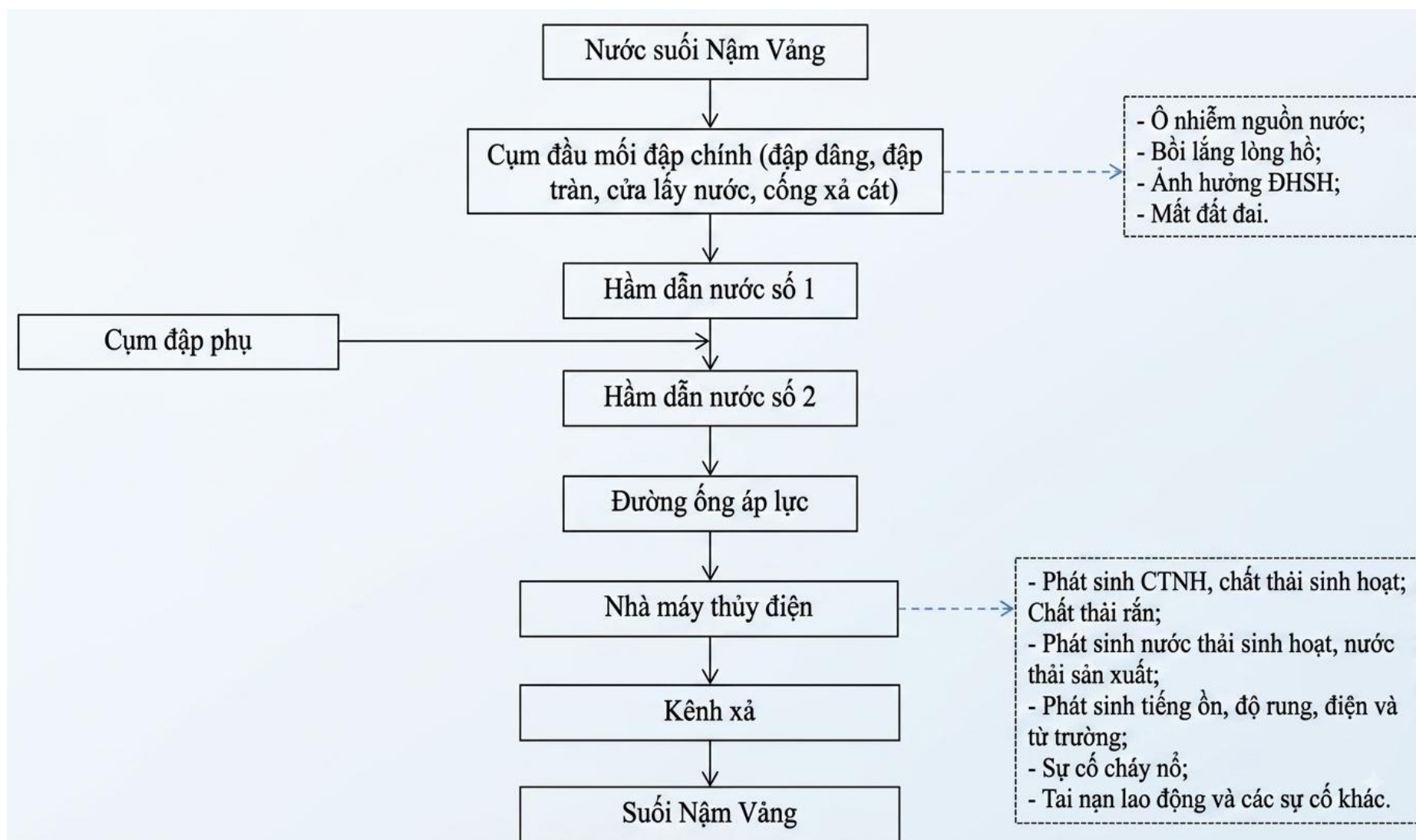
Hình 1. 1. Sơ đồ quy trình vận hành sản xuất Dự án thủy điện Nậm Ban 1A
