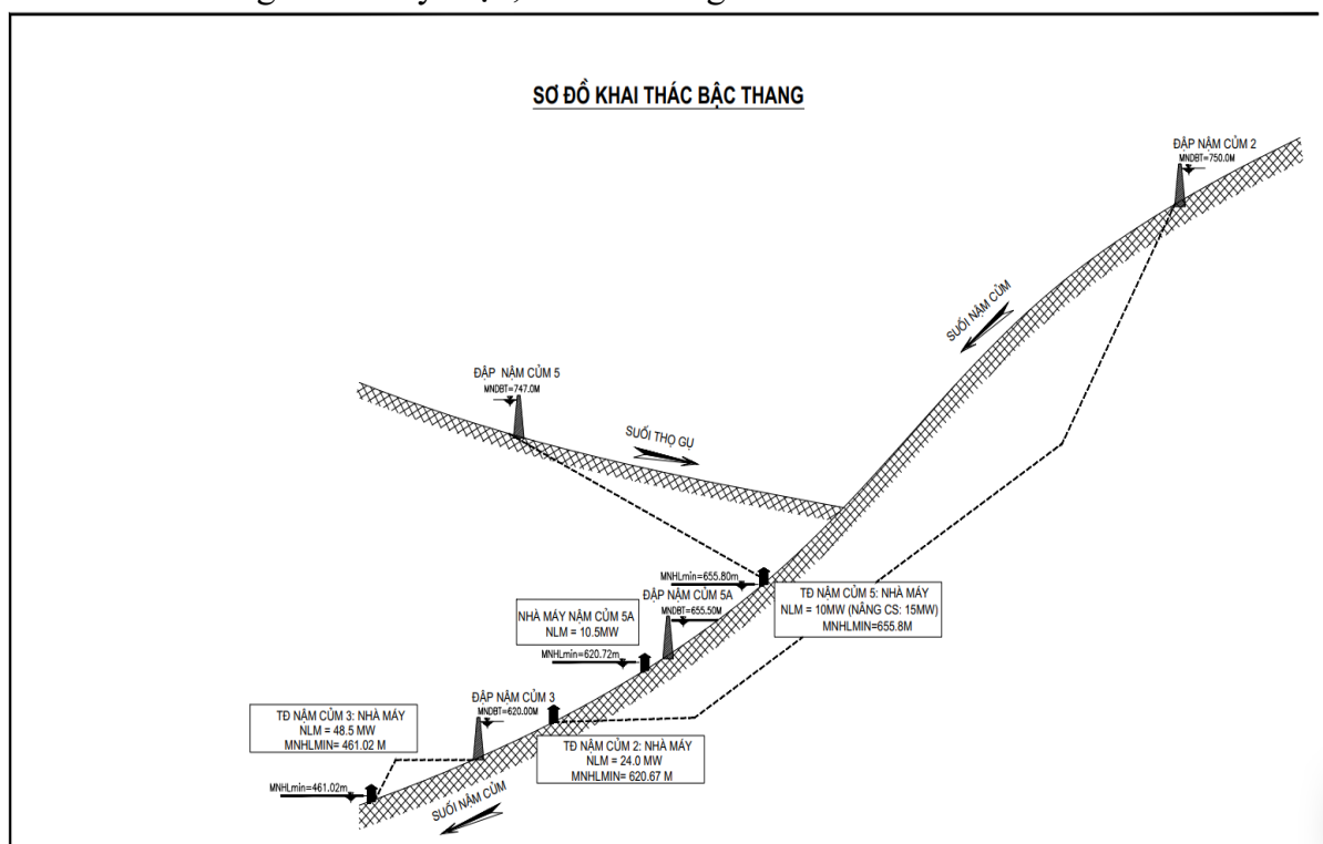
Hình 0. 1. Mối liên hệ quy hoạch thủy điện trên suối Nậm Cúm
