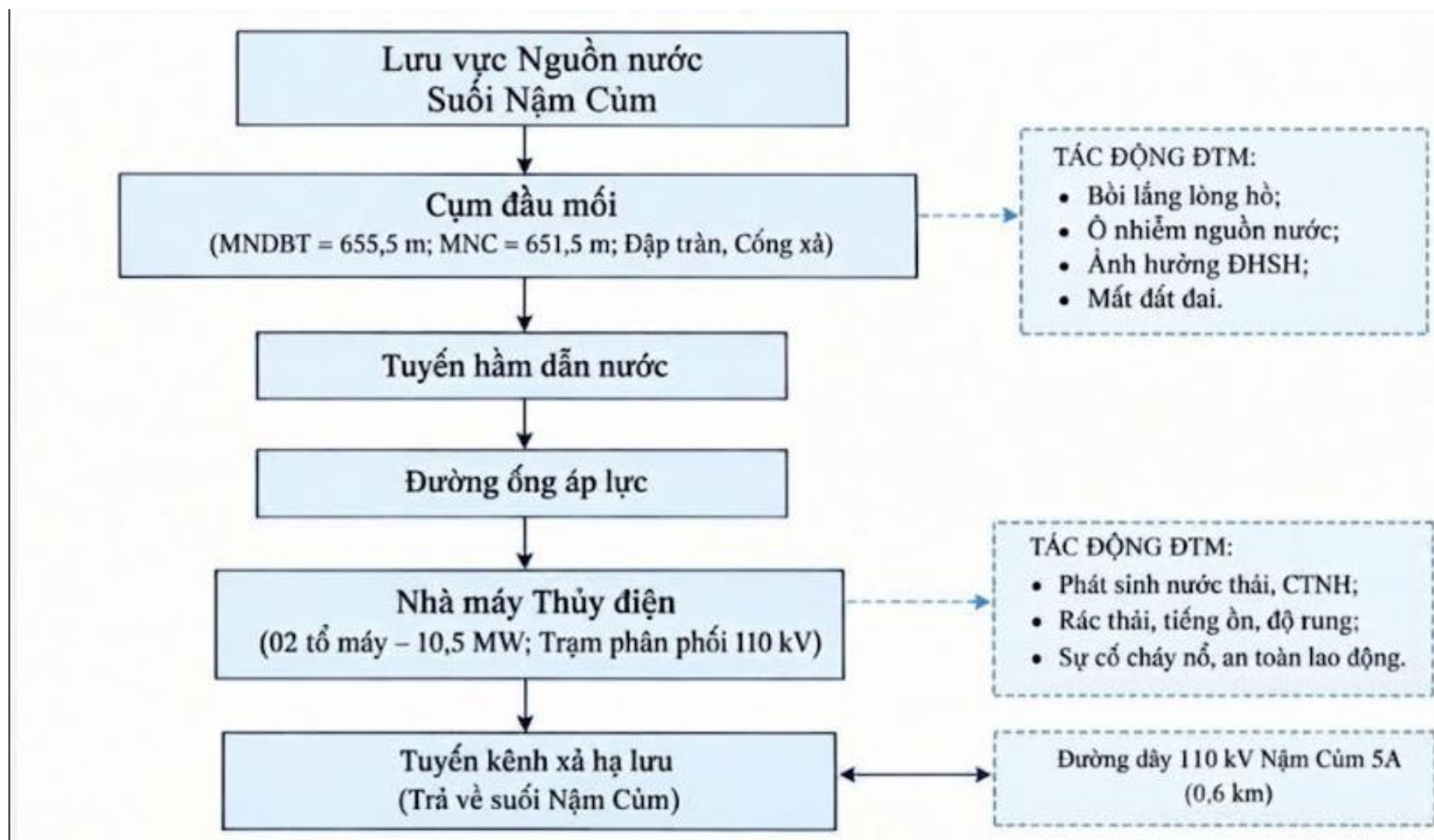
Hình 1. 1. Sơ đồ quy trình vận hành sản xuất Dự án thủy điện Nậm Cùm 5A
