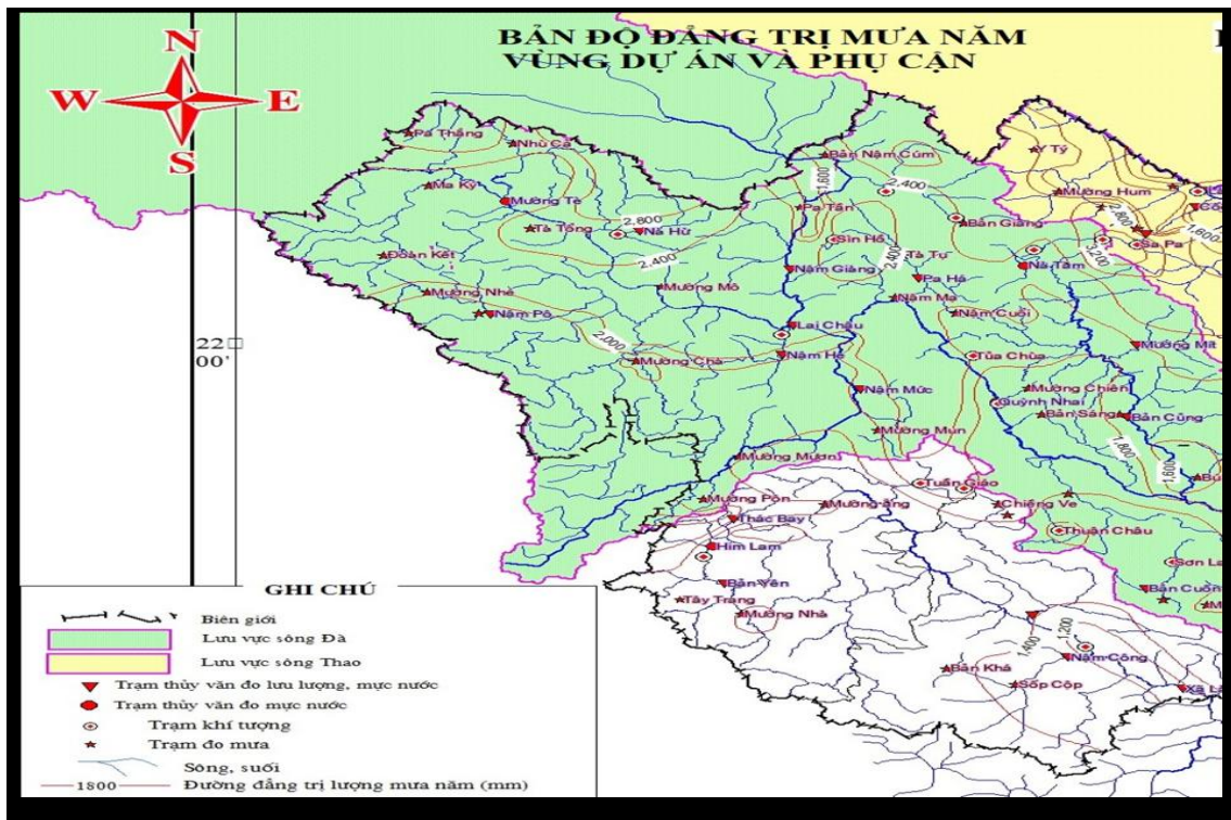
Hình 2. 1. Vị trí các trạm khí tượng, thủy văn và bản đồ đẳng trị mưa khu vực dự án thủy điện Nậm Cúm 5A
