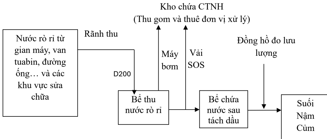
Hình 3. 2. Sơ đồ quy trình xử lý nước nhiễm dầu
