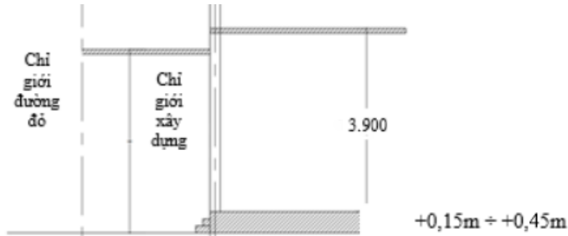
Hình 5. Quy định về chiều cao công trình và cốt nền công trình
