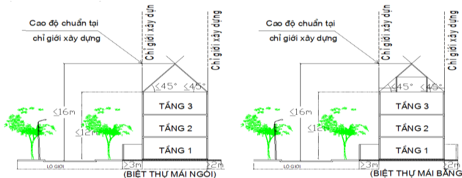
Hình 3. Quy định tầng cao, chiều cao đối với nhà vườn, biệt thự
